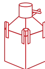
Boca Cónica con tapa
